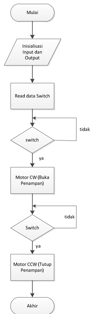
Gambar 6. Diagram Alir Motor Pada APGD
