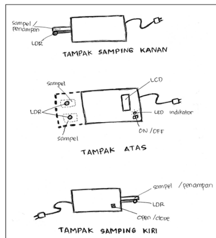
Gambar 2. Sket Desain Alat
